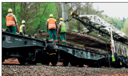
Vozový jeřáb UK 25/18 vytrhává kolejová pole za sebou a nakládá před sebe na speciální plošinové vozy, tzv. rolničky. Foto: Petr Buryška
